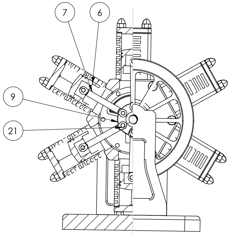
SECTION A-A SCALE 1 : 3
