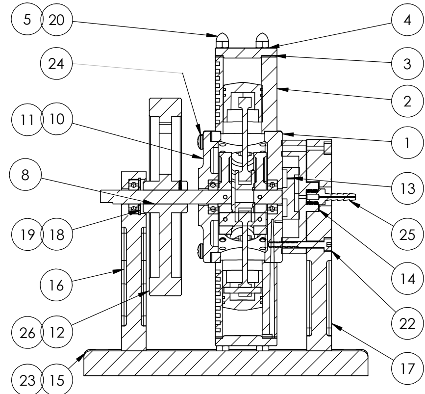
SECTION B-B SCALE 1 : 3
